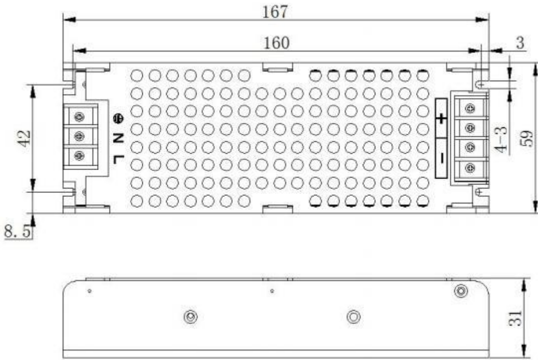
d. CL-AS11-200-5D 外形尺寸
