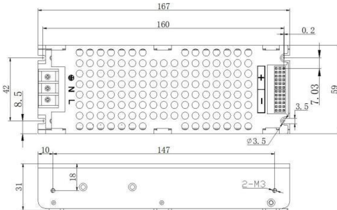
d. CL-AS11-200-5D 外形尺寸
